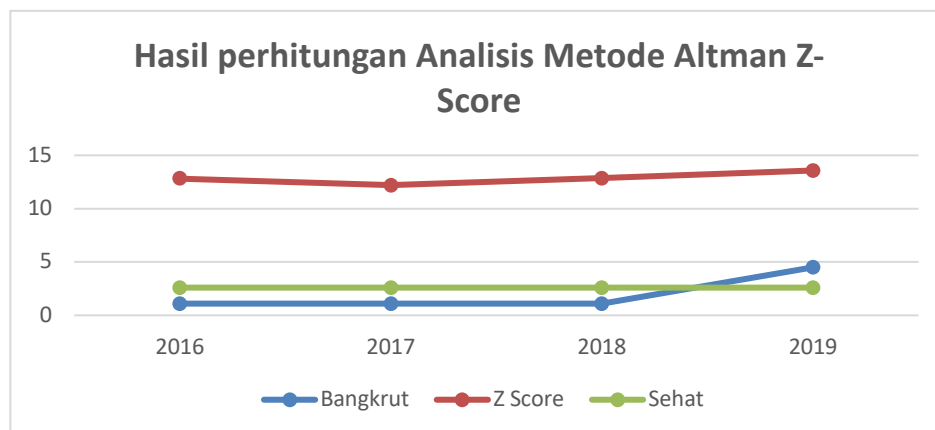
Gambar 1. Grafik Metode Altman Z-Score
